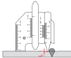
derinlik ölçümü
